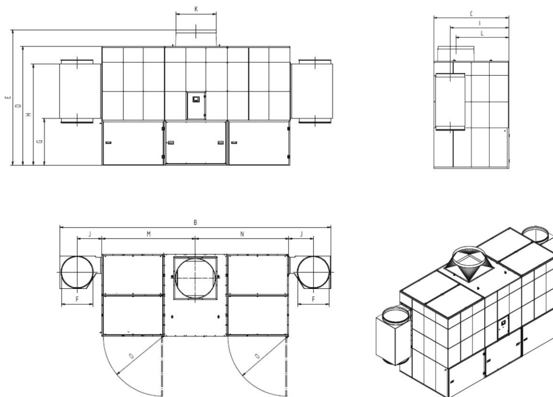
Fig. 79: Folha de dimensões 34200 + 34220
