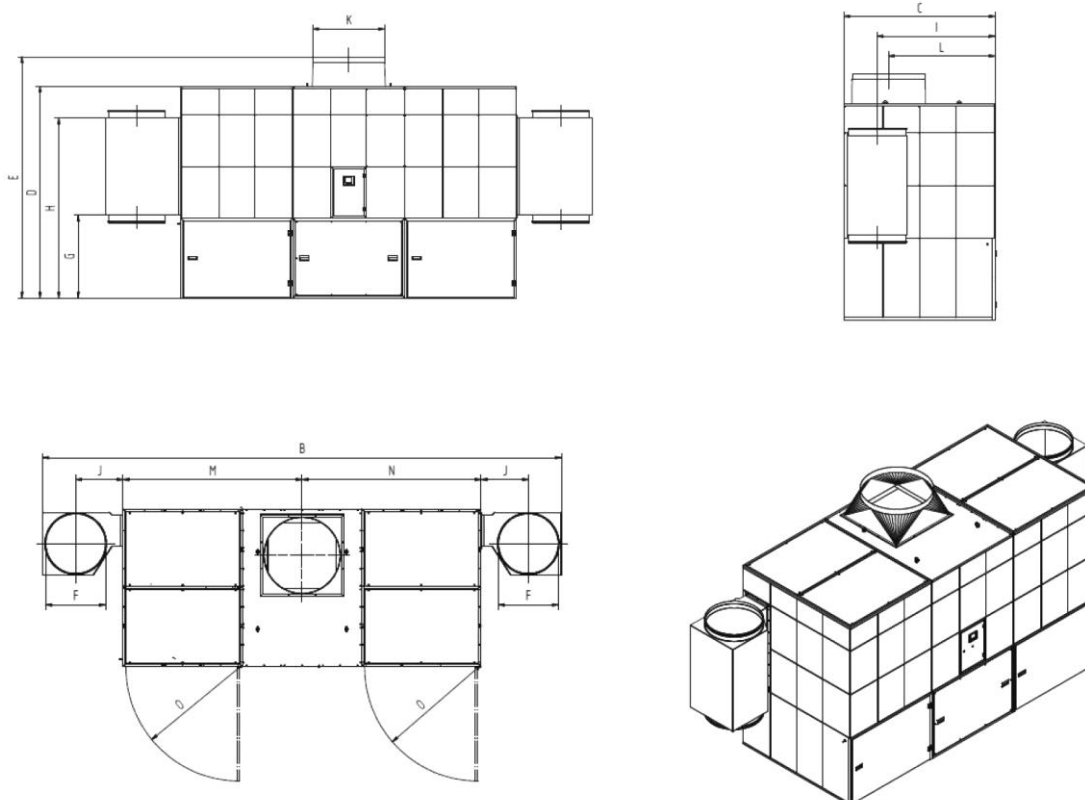
Fig. 78: Folha de dimensões 34180
