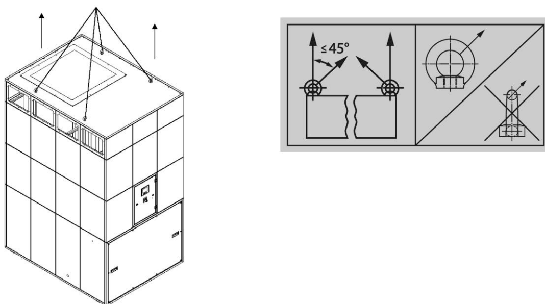
Fig. 18: Elevação do filtro com grua
