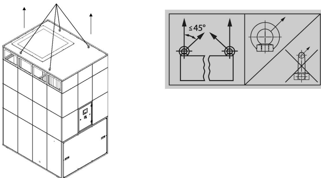
Fig. 10: Elevação do ventilador com grua
