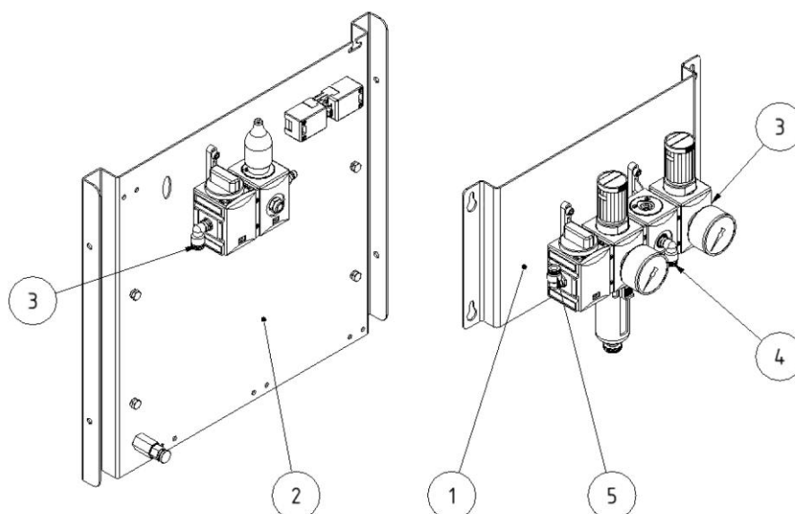
Fig. 31: Unidade de ar comprimido
