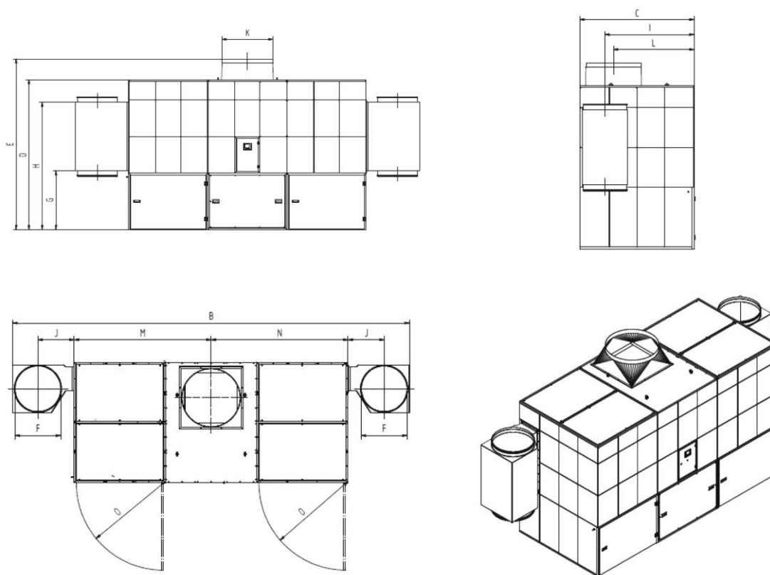
Fig. 77: Folha de dimensões 34160
