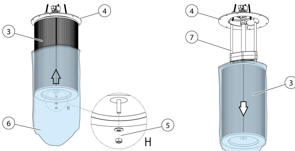
Fig. 68: Substituição do filtro– desmontar o cartucho do filtro
