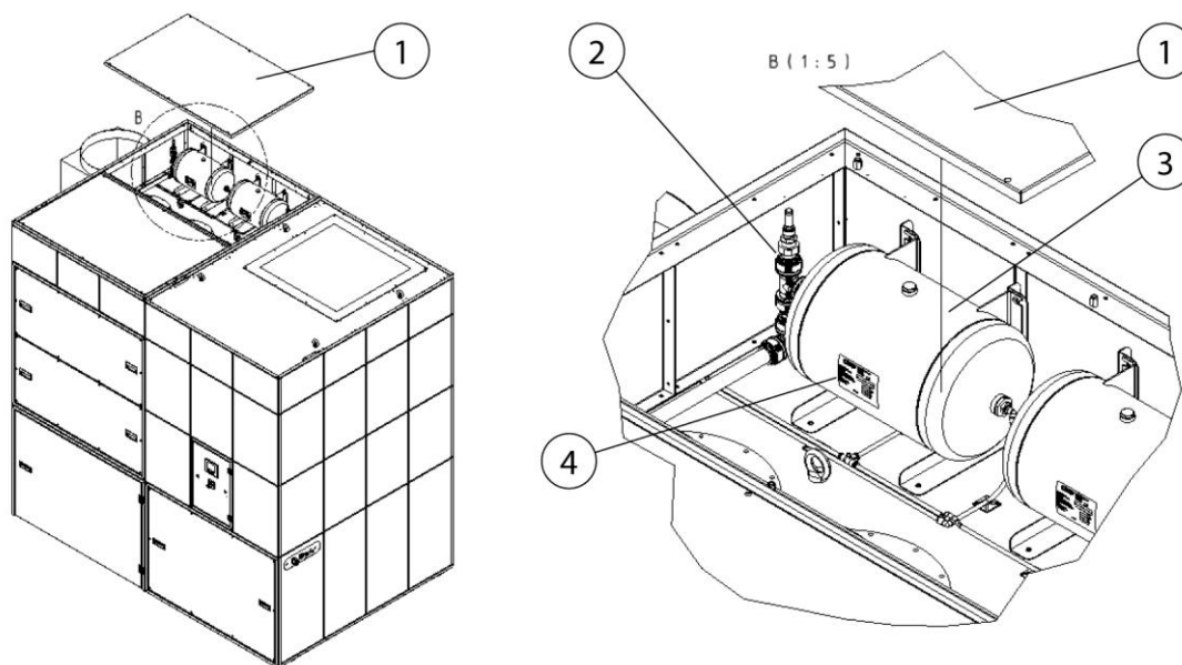
Fig. 74: Acesso ao reservatório de ar comprimido + válvula de segurança
