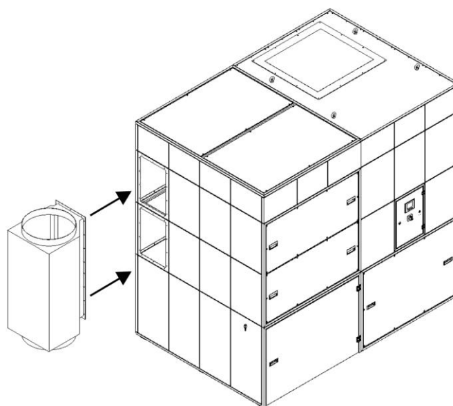
Fig. 26: Montagem da caixa de ligação do lado da aspiração
