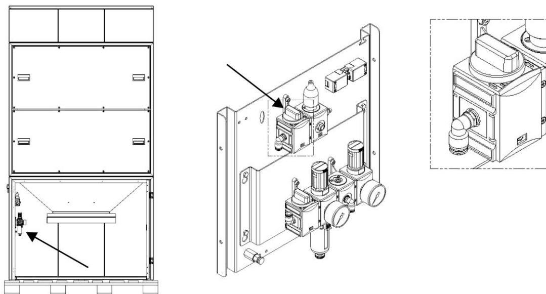
Fig. 14: Válvula de abaixamento recipiente coletor de pó
