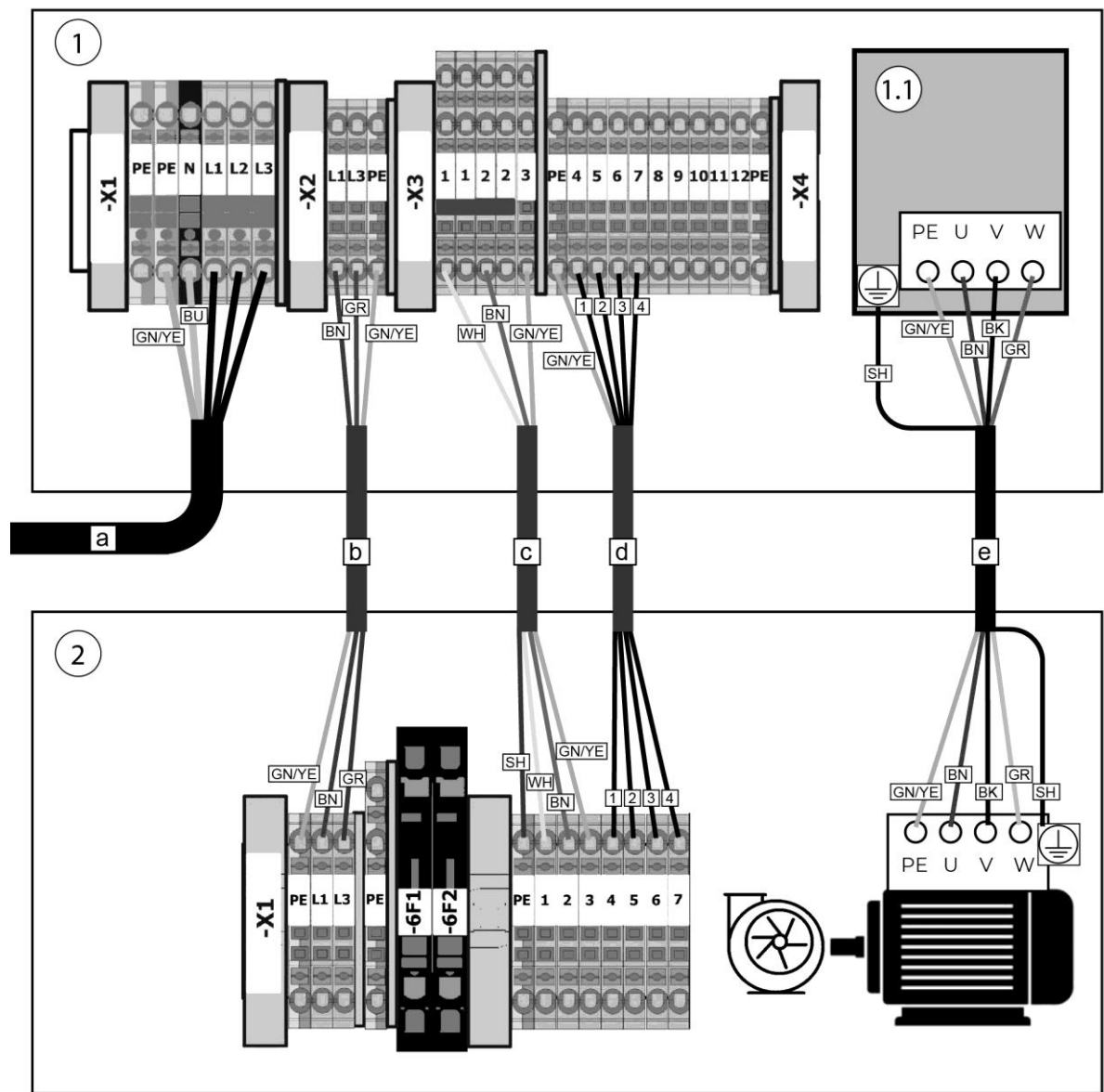
Fig. 35: Esquema de cablagem da regulação da potência de aspiração com produto
