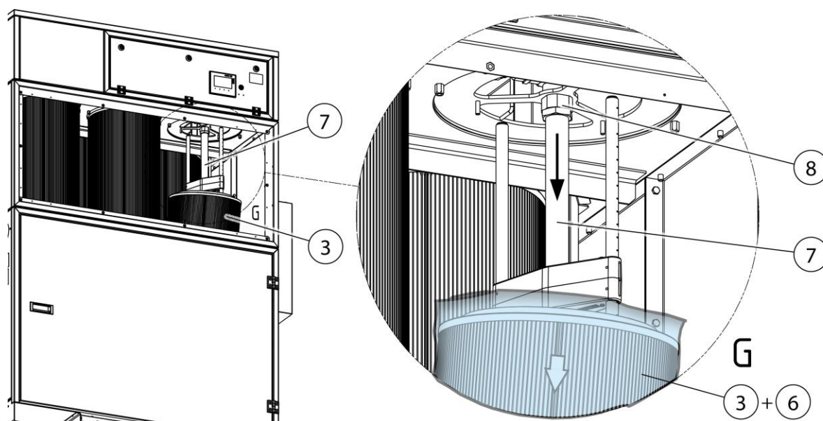
Fig. 63: Desmontar bico giratório
