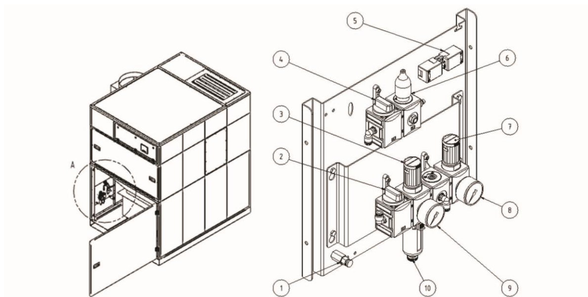
Fig. 27: Unidade de ar comprimido
