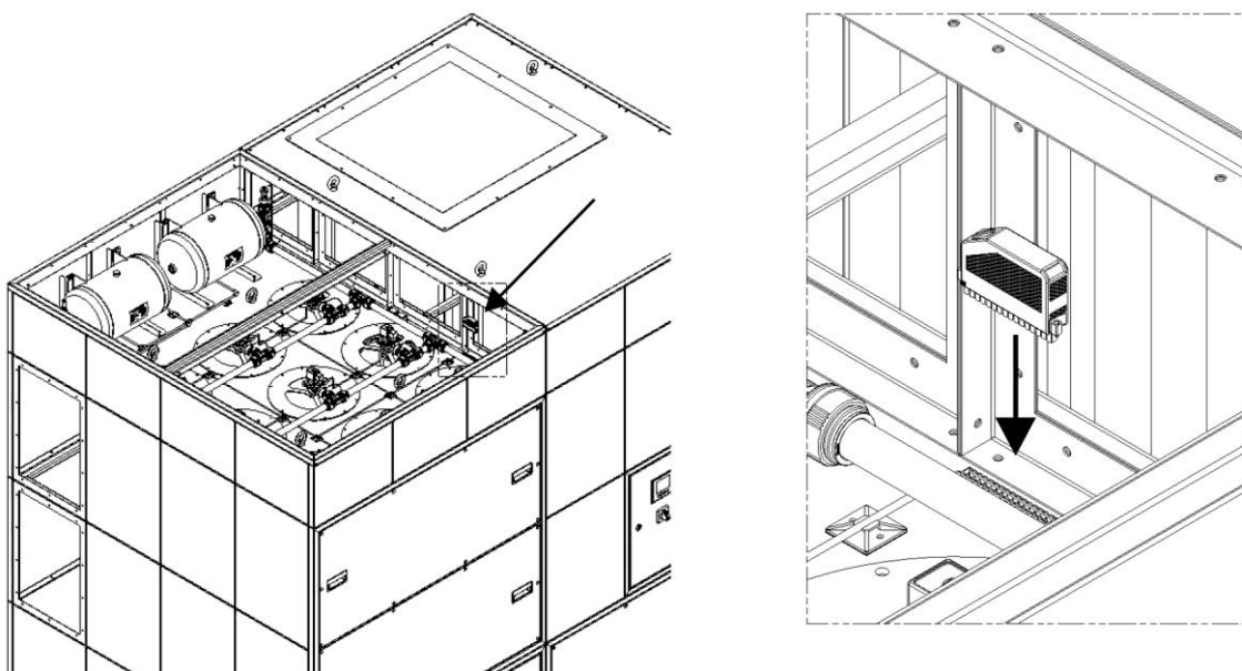
Fig. 22: Montagem da ficha verde
