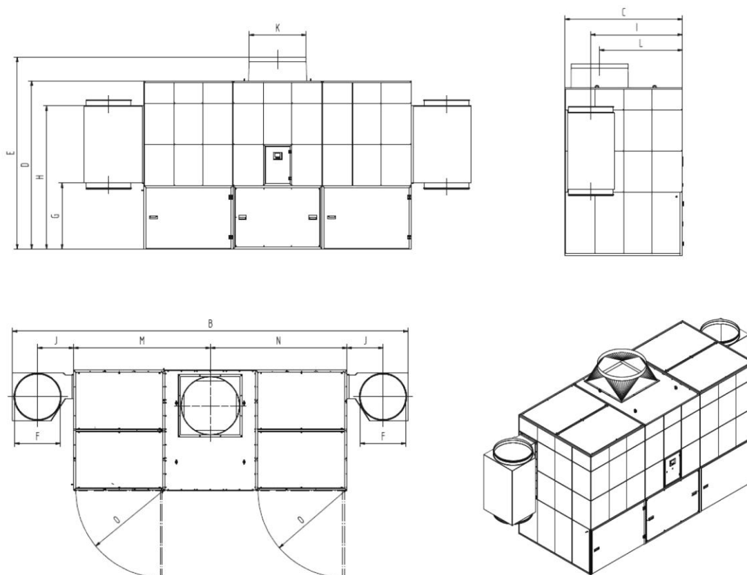
Fig. 80: Folha de dimensões 34240 + 34270
