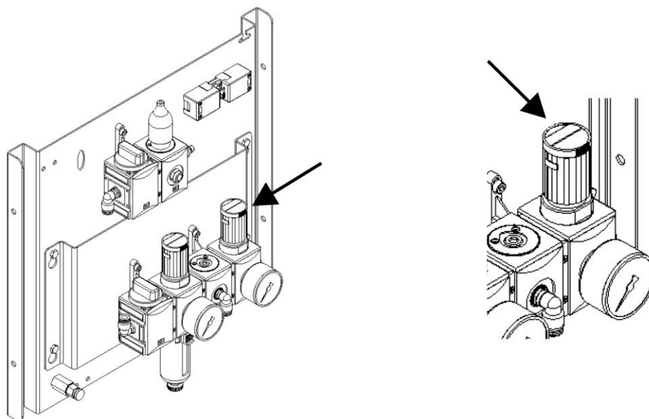
Fig. 30: Ajuste da pressão do dispositivo de elevação/recipiente coletor de pó
