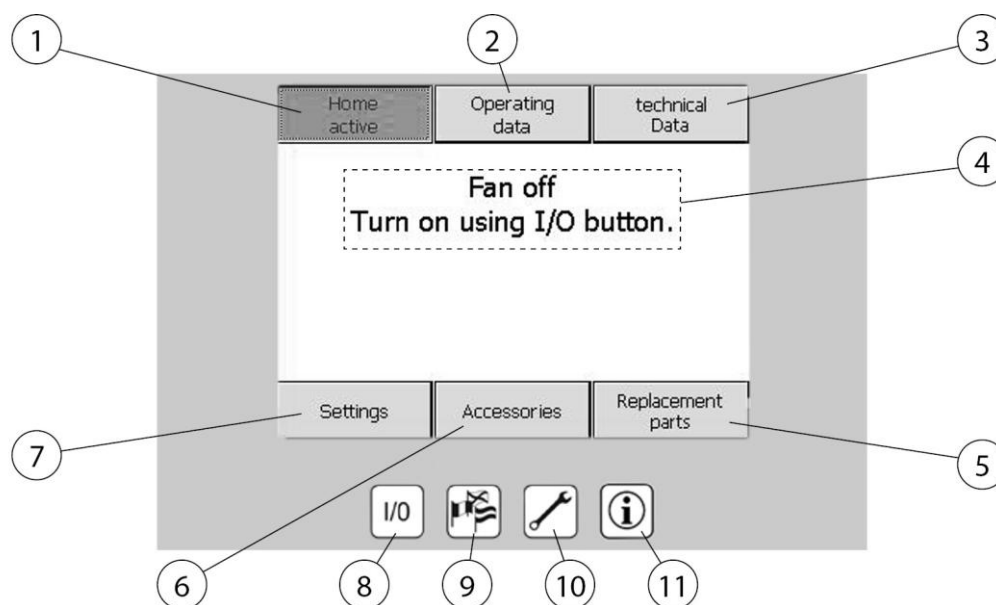
Fig. 38: Elementos de comando
