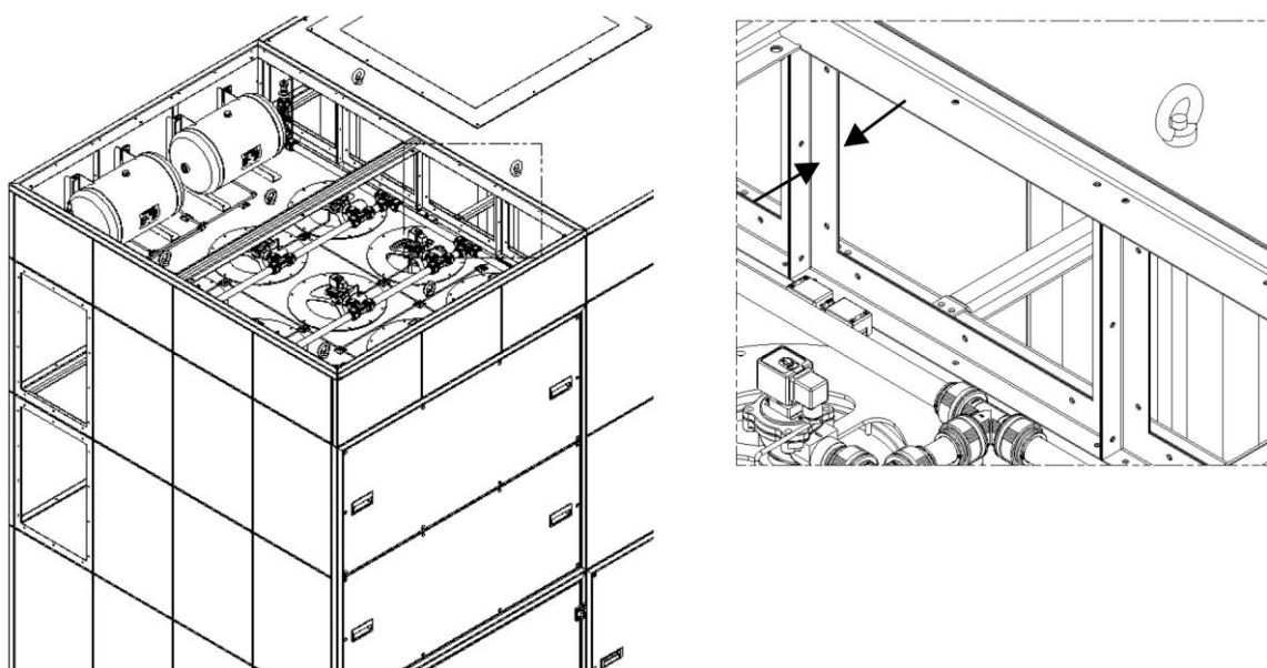
Fig. 21: Unir o ventilador ao filtro
