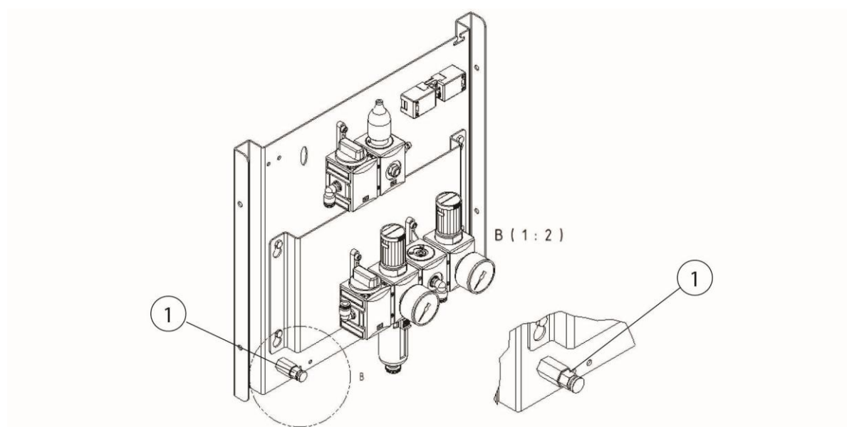
Fig. 70: Válvula de drenagem de condensado do reservatório de ar comprimido
