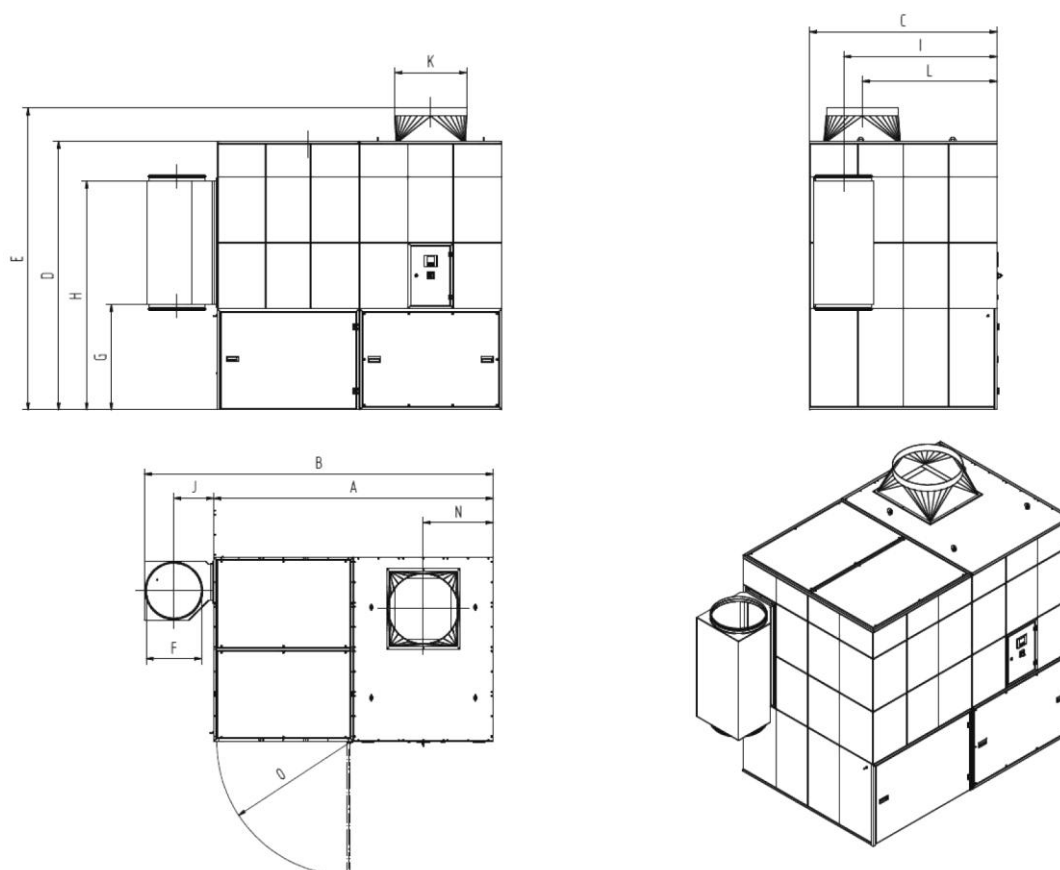
Fig. 76: Folha de dimensões 34130
